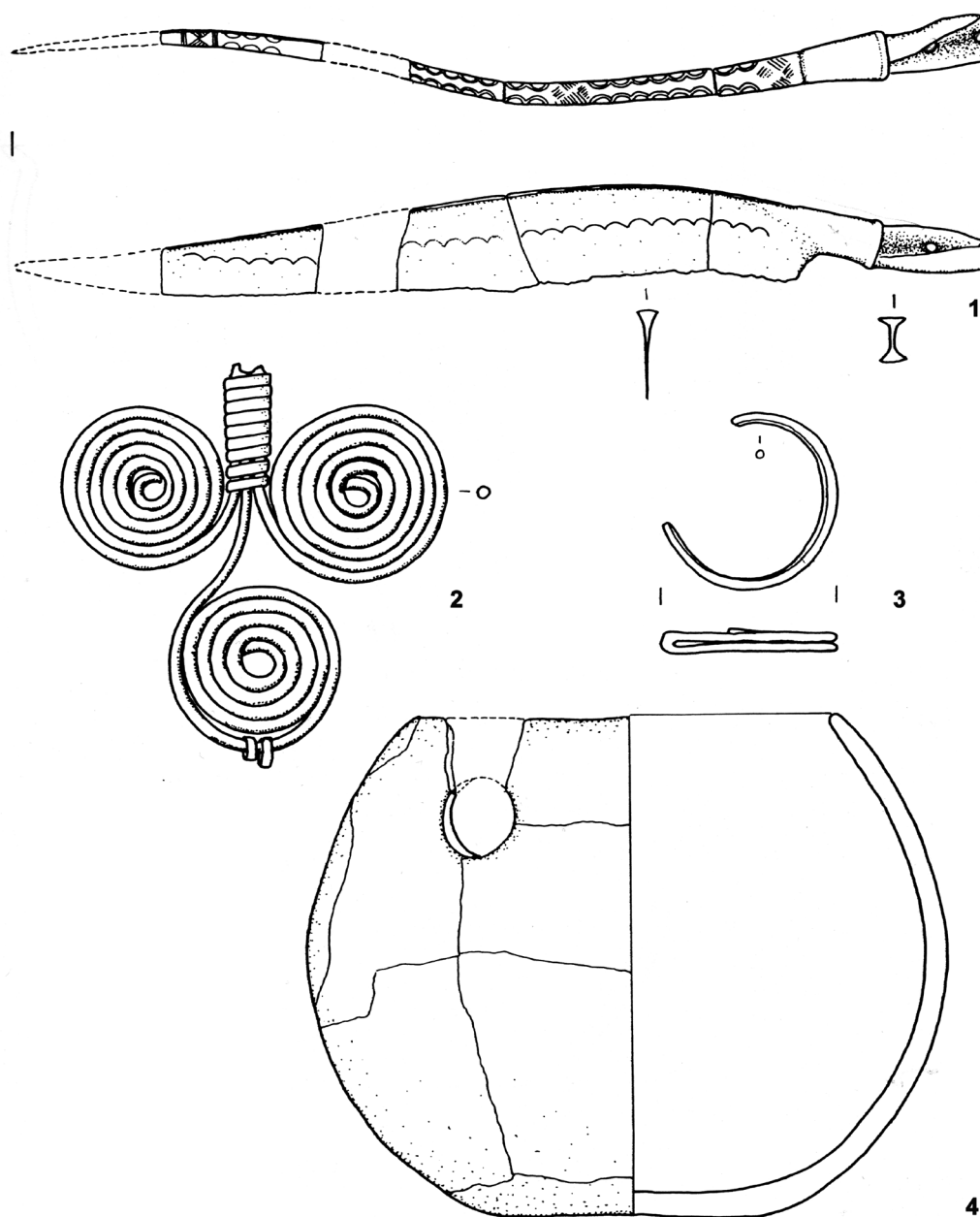
Sl. 3 – Inventar groba 4/1911 iz nekropole u Velikoj Gorici (prema Karavanić 2009, T. 63).
