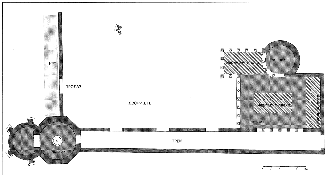
12. Медијана, hipotetičanstavljena реконструкција истраженог дела виле са октогоном (према Г. Милошевић)
