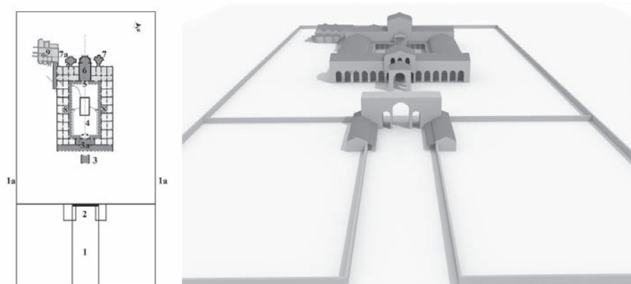
Sl.6 Mediana, kompleks vile sa peristilom, II graditeljska faza, osnova i idealna rekonstrukcija akroz monumentalnu antičku kapiju u izgledu slavluka: 1) prilazni svečani put; 1a) ogradni zid; 2) antička kapija (G. Milošević)
