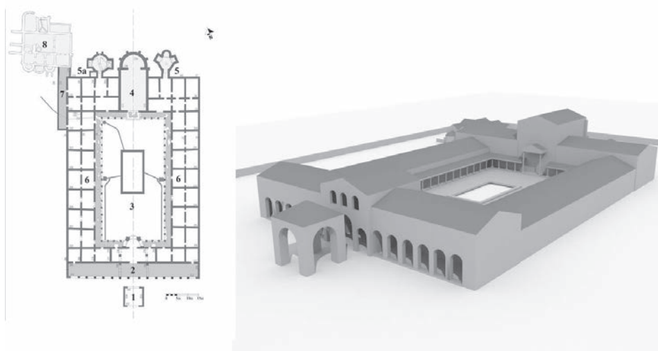
Sl. 5. Mediana, vila sa peristilom, II graditeljska faza, osnova i idealna rekonstrukcija: 1) vestibul; 2) južni trem i prostorije za potrebe predstavljanja ( salutatorium ) i čekanja; 3) peristil; 4) sale za audijenciju ( consitorium ) i banket ( trichorum ); 5-5a) stibadium; 6) officium ; 7) hodnik prema termama; 8) terme (G. Milošević)
