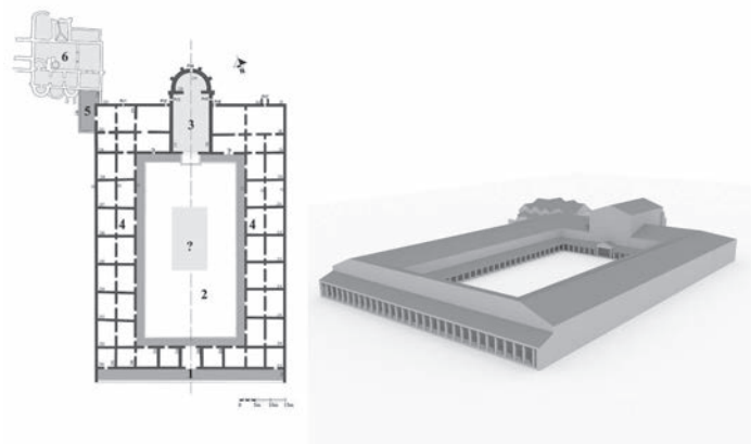
Sl. 4. Mediana, građevina sa dvorištem, I graditeljska faza, osnova i idealna rekonstrukcija: 1) trem; 2) dvorište sa tremom; 3) aula; 4) officium (G. Milošević)
