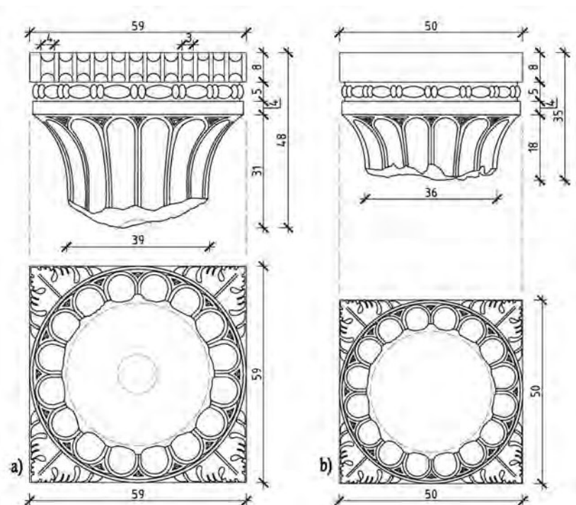
Сл. 2 Велики (а) и мали (б) канелирани палмин капител у Архео-етно парку у селу Равни (изгледи и основе)
