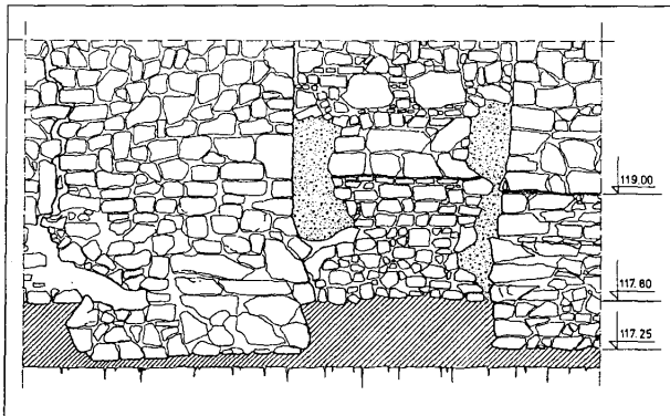
Сл. 10 - Сонда 2/72 - изглед лица зида са темељом куле V. Fig. 10 - Trench 2/72 - outer face of the wall with foundation of tower V.
