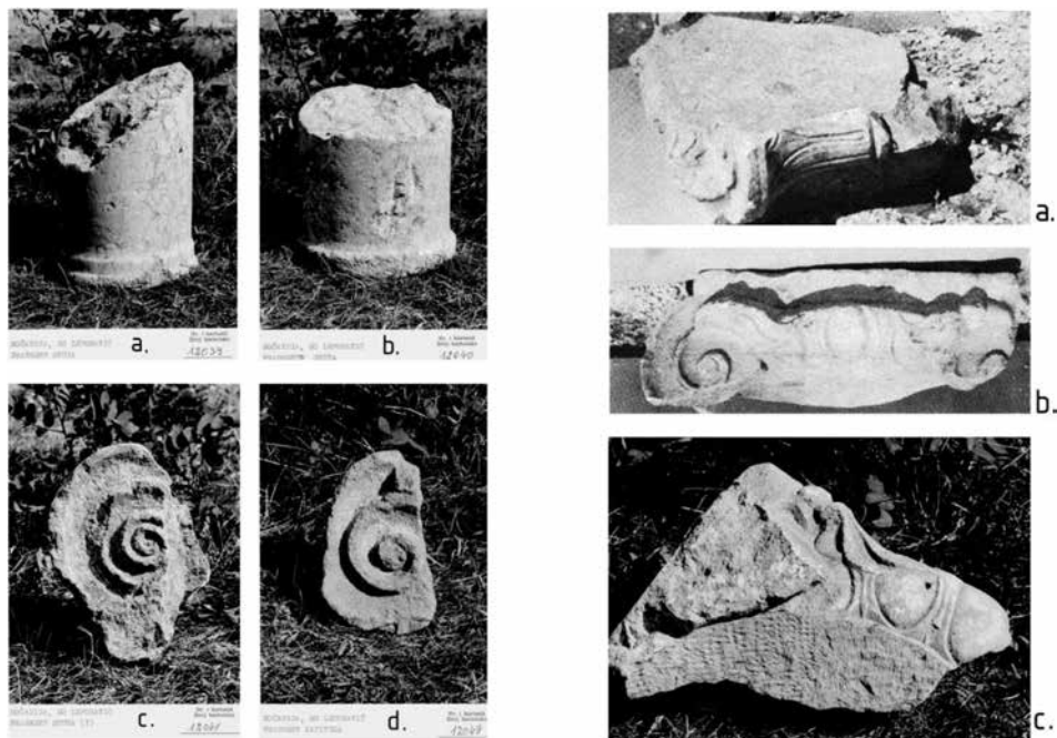
Сл. 2. Фотографије делова стубова: (лево) а. и б. стабла пречника 15 см; с. и д. Обијене волуте са јонских капитела пронађене на простору форума (Документација РЗЗСК у Београду); (десно) фотографије јонских капитела пронађених на простору форума: а. и б. Објављено у дисертацији Емила Чершкова (Čerškov 1970: TVI.2,3) и с. четвртина капитела из документације РЗЗСК у Београду.
