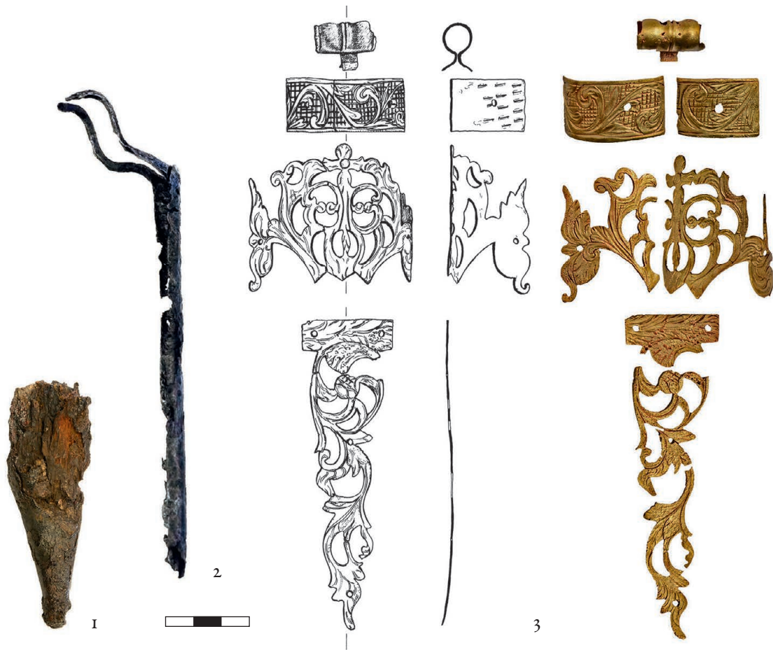
Сл. 89. Налази наоружања: каније сабљи (Документација Археолошког института)
