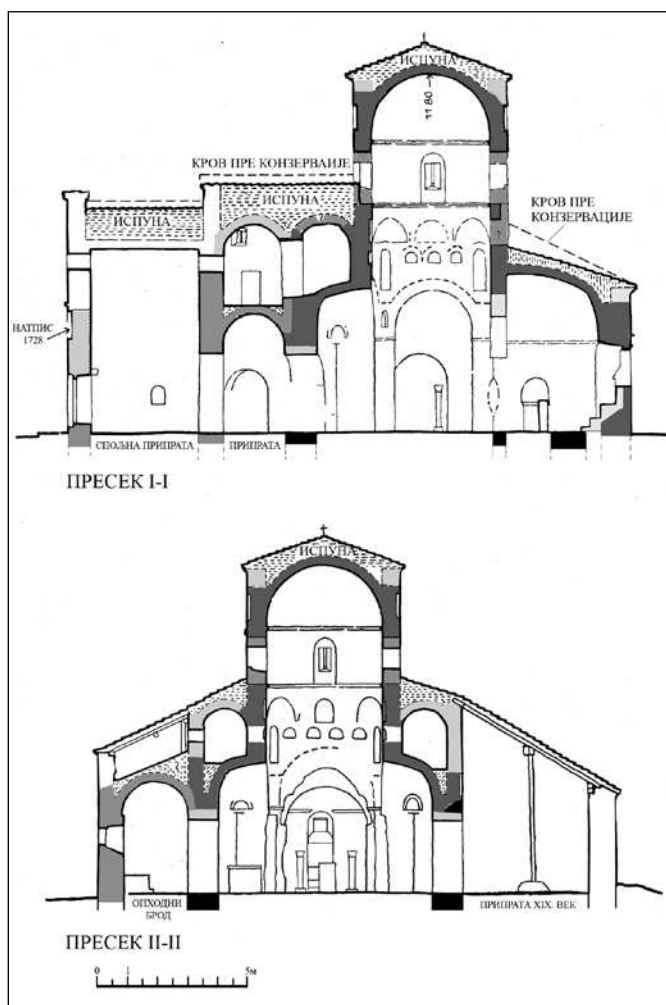
Сл. 2а Подужни пресеци Цркве св. апостола Петра и Павла код Новог Пазара према Ј. Нешковић, Петрова црква код Новог Пазара , 7, 9, план 3, 4, са изменама.
