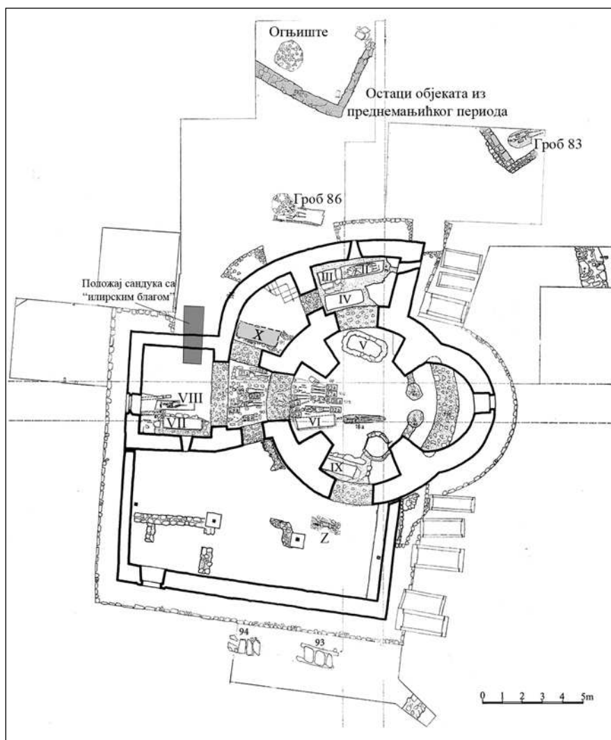
Сл. 3 Основа Цркве св. апостола Петра и Павла код Новог Пазара према М. Љубинковић, Некропола цркве св. Петра код Новог Пазара , комбиновани подаци са планова 2, 3, 4.
