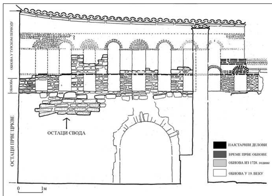
Сл. 4 Кружни зид цркве на јужној страни (развијена дужина) према Ј. Нешковић, Петрова црква код Новог Пазара , 20, слика 16.
