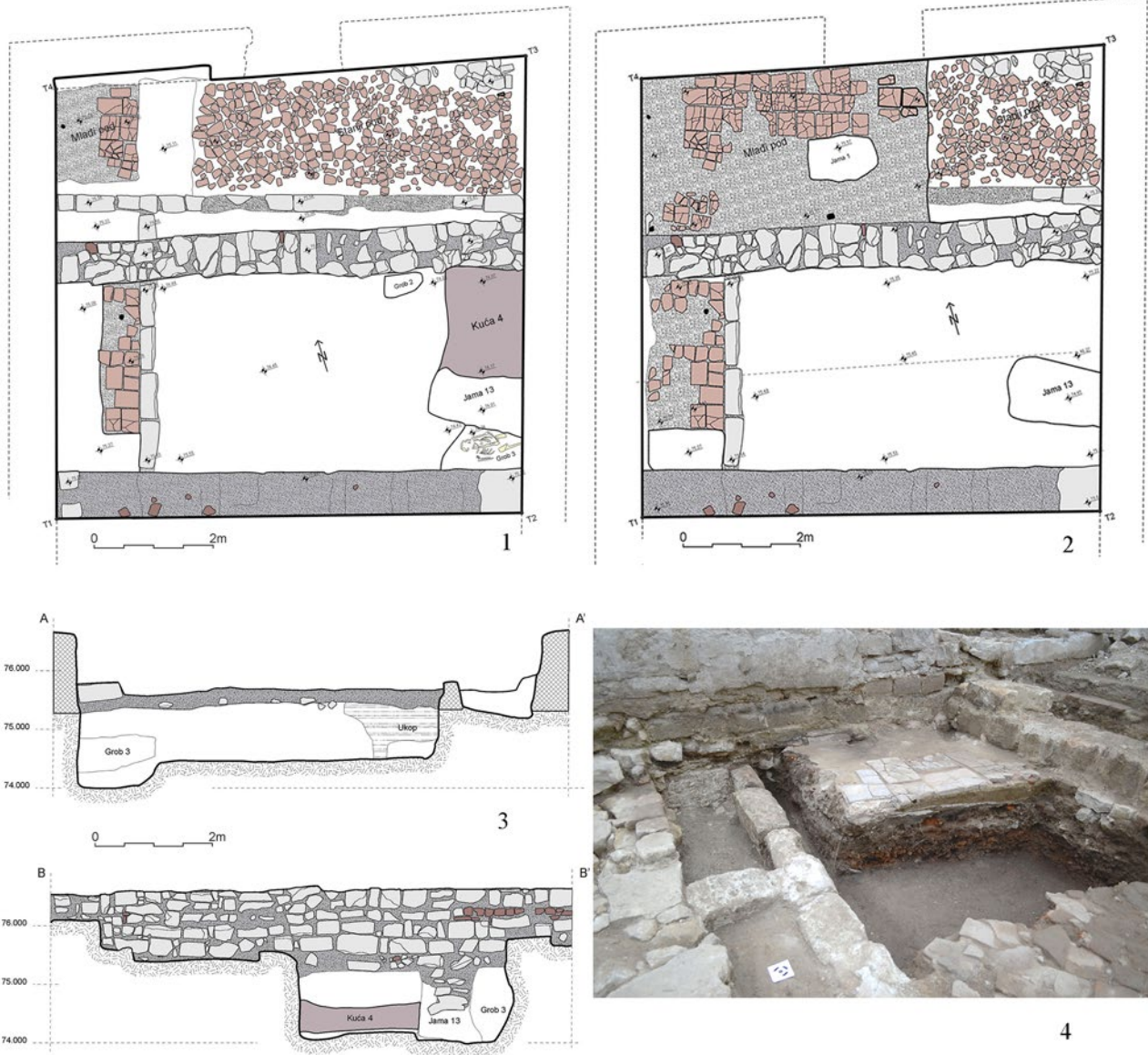
Сл. 12. Осџаци објеката XVI–XVII века (извор: Документација Археолошкој институције)
