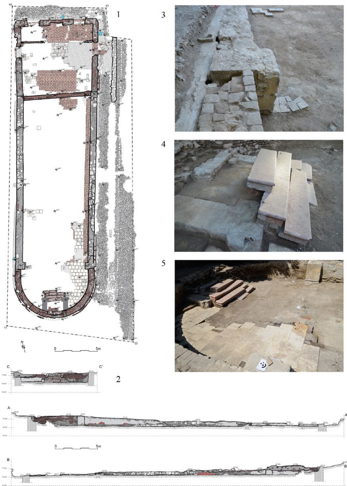
Сл. 18. Синаіоіа у њрећој фази: 1) основа; 2) ѡресеци зигова; 3-5) деѡаљи айсиде и ѡиластѡра (извор: Документѡација Археолошкој инстѡиѡуѡи)
