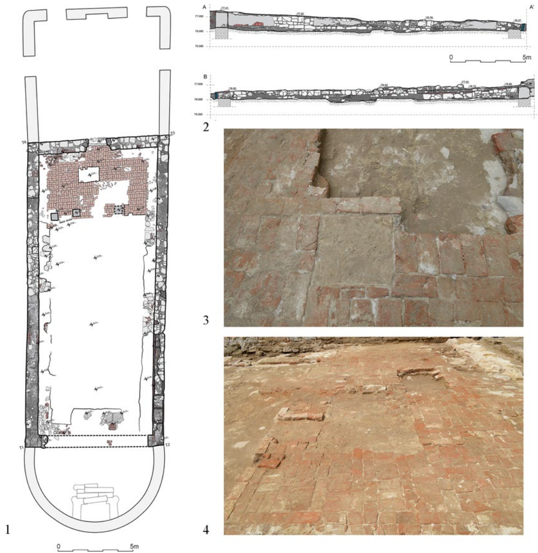
Сл. 16. Синагога у другој фази: 1) основа; 2) пресеци зидова; 3–4) детаљи једног зидова и база стубова (извор: Документација Археолошкој институције)
